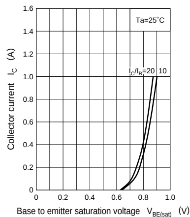
I_C - V_{BE(sat)}
