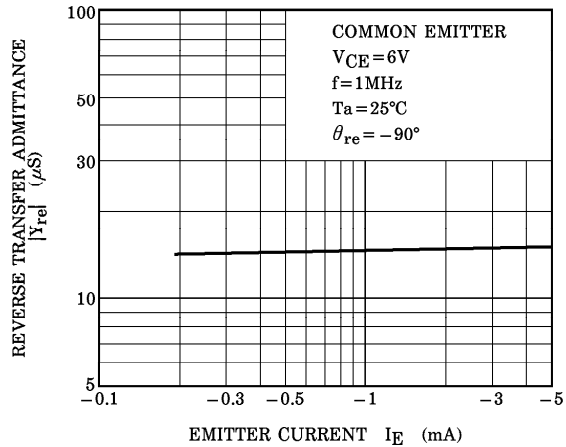
|Y_{re}| - I_E
