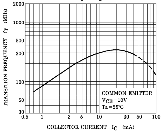
f_T - I_C
